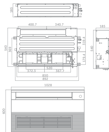
AB25 - AB35 - AB50 - AB71
